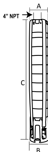
Acoplamiento NEMA 4" Fig. 1
