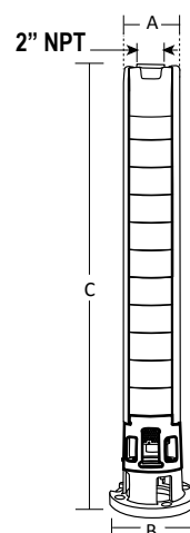
Acoplamiento NEMA 4"
